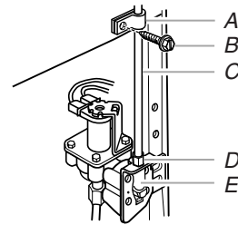
A. Bride du tube D. Écrou de compression B. Vis de bride du tube E. Entrée du robinet C. Tube en plastique
