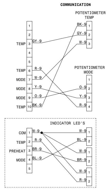
SINGLE WALL OVEN CIRCUIT // CIRCUITO DEL HORNO DOBLE // CIRCUIT DU FOUR DOUBLE
